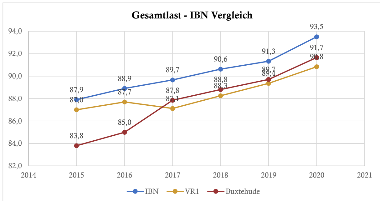
Abbildung 5: Gesamtlast - IBN Vergleich
