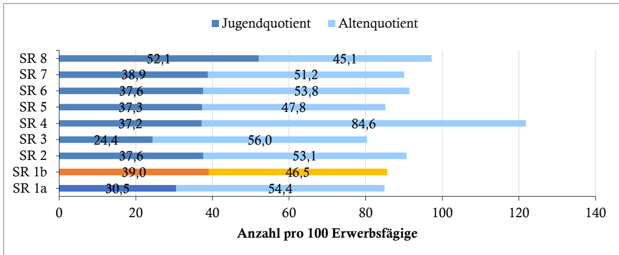
Abbildung 129: Gesamtlast SR 1b
